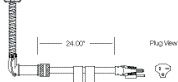
Fuente de alimentación de 90 Grados con clavija de 20A. BE42135-3-1-90-ST_XX
