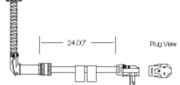
Fuente de alimentación de 90° con clavija de angulo de 90° de 20 Amp. BE42135-3-1-90-RA_XX
